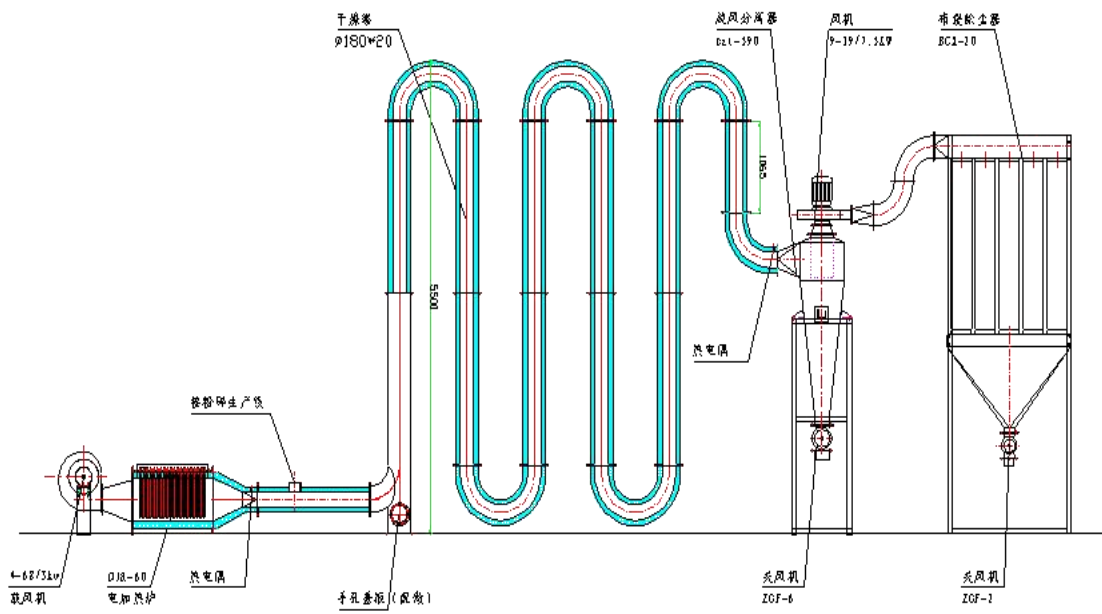
立面布置图
