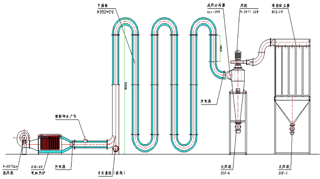
立面布置图
